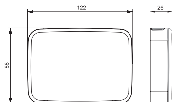
Sonde AIRSENS
