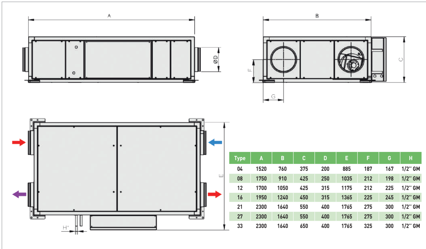
CADB/T-HE 04 à 33 LH/RH
