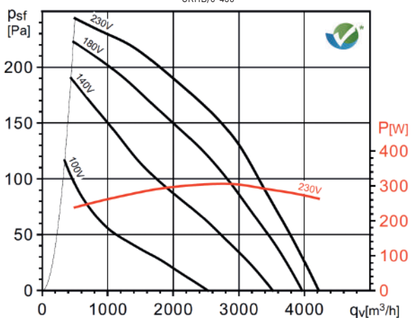
CRHB/6-450
