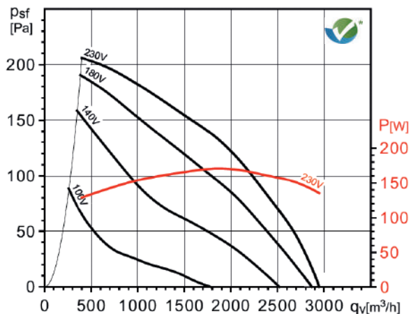
CRHB/6-400
