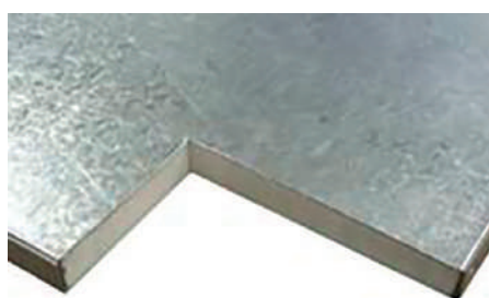
Isolation double-peau par 25mm de laine de verre ininflammable
