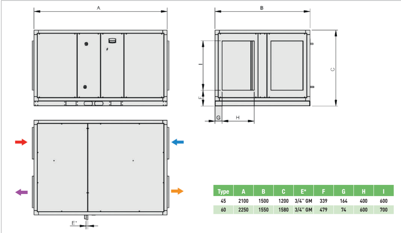
CADB/T-HE 45 et 60 LH/RH
