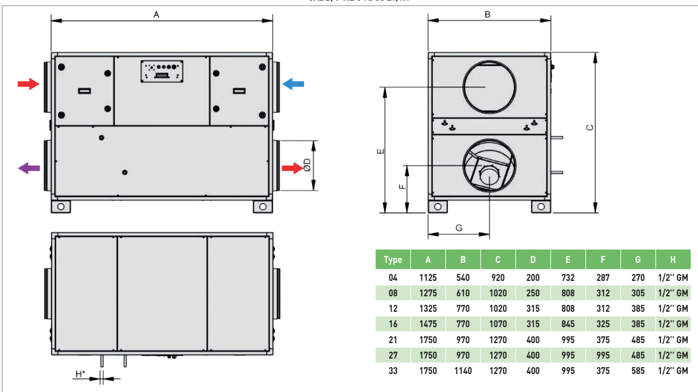
CADB/T-HE 04 à 33 LV/RV
