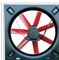
Configuration de construction modèles Ø 800 à 1000 mm
