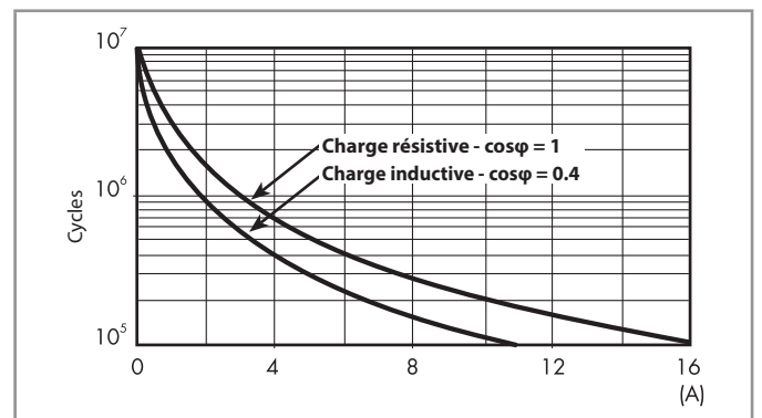
F 46 - Durée de vie électrique (AC) en fonction de la charge
