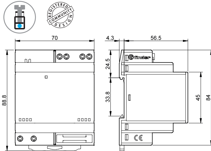
Types 78.51 / 78.61 Bornes à cage
