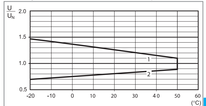
R 22 - Plage de fonctionnement en fonction de la température ambiante
