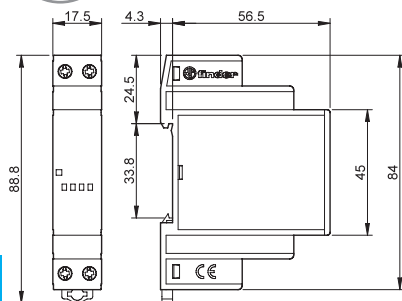
77.01 DC Bornes à cage
