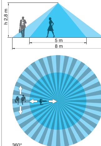
18.31...0031 - Installation sous plafond grande hauteur
