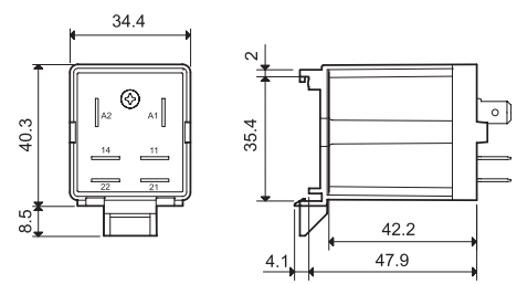
065.07 avec relais monté
