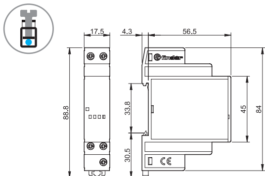
Type 19.91 Bornes à cage
