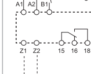
Schéma de raccordement (avec Signal de commande)
