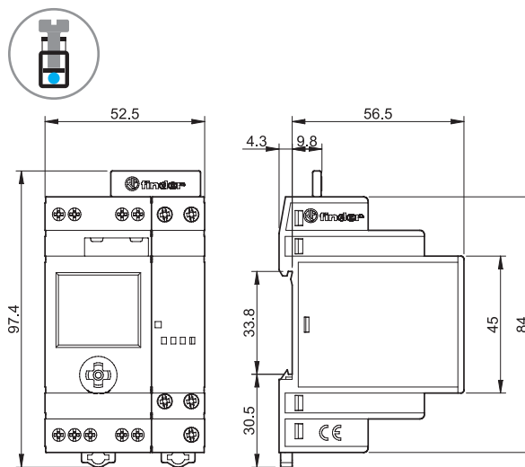
11.91 + module de puissance 19.91 Bornes à cage
