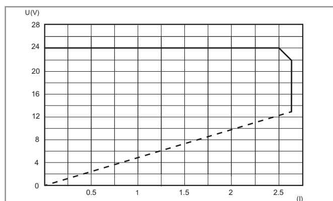
FB78-2 Tension de sortie en fonction du courant de sortie (78.61)
