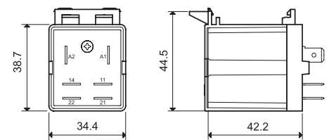
065.08 avec relais monté
