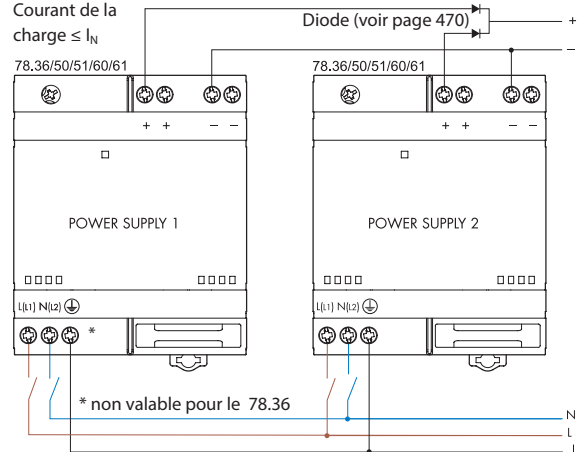
Connexion redondante manuelle
