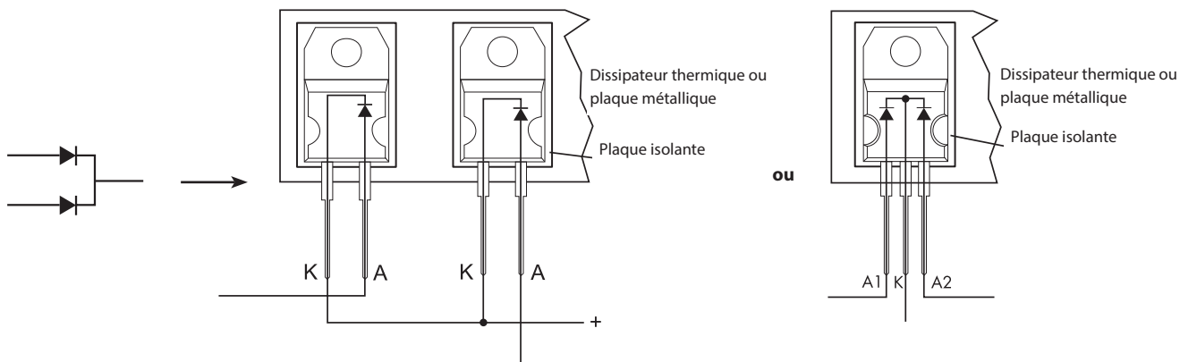
Diode pour type 78.25, 78.36, 78.50, 78.60, 78.51, 78.61
