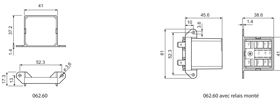
062.60 avec relais monté
