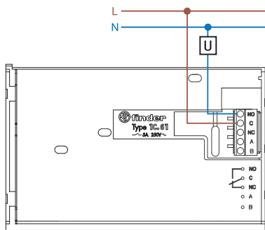
Schéma électrique
