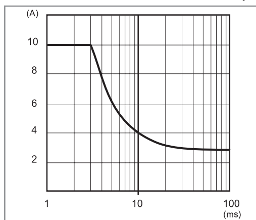
P78-5 Pic de courant en sortie en fonction du temps (78.50/51)
