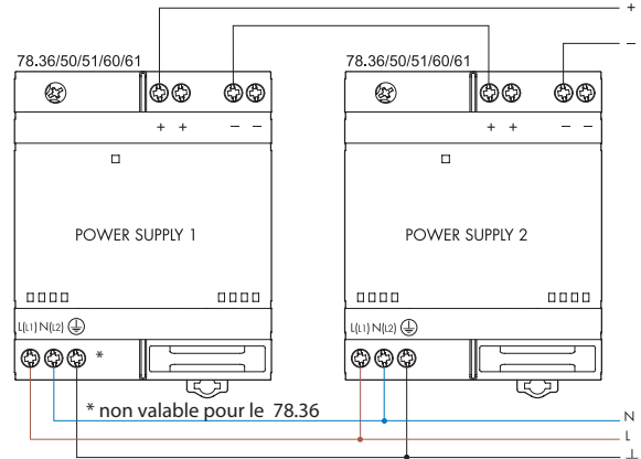
Raccordement en série
