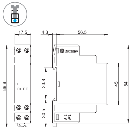
13.81 Bornes à cage
