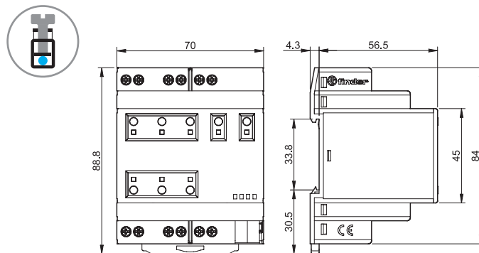
Type 19.6K Bornes à cage
