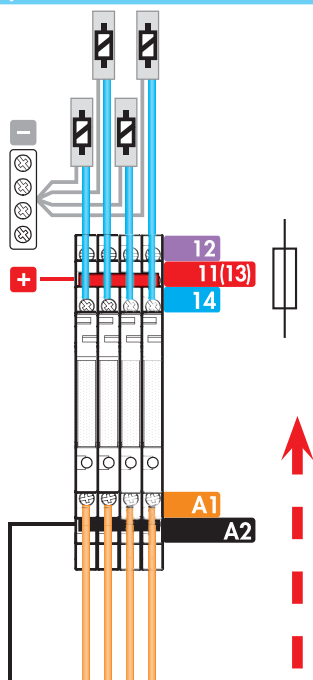
Sortie automate
