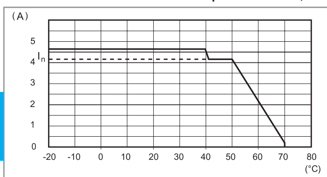
L78-5 Courant de sortie en fonction de la température ambiante (78.50/51)
