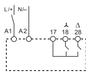
Schéma de raccordement (sans Signal de commande)
