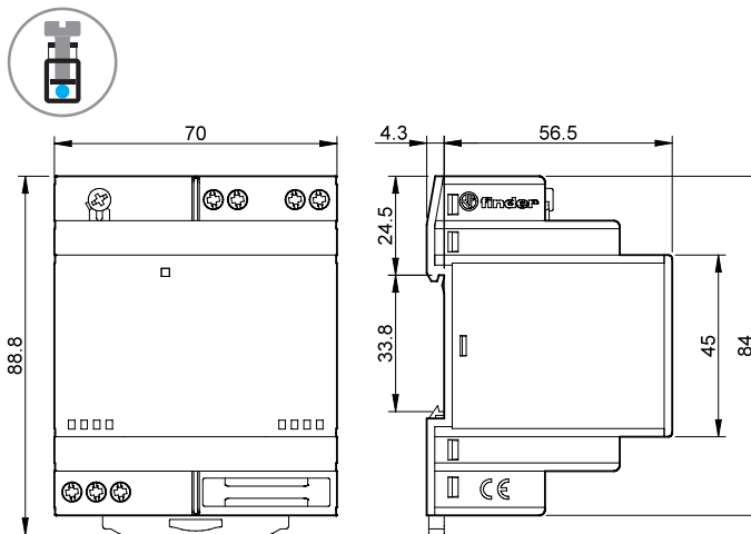
Types 78.51 / 78.61 Bornes à cage
