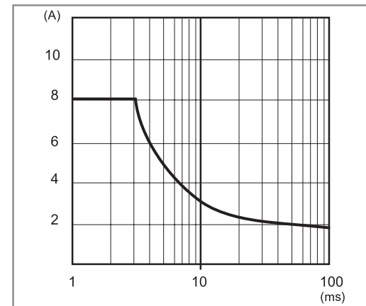
P78-2 Pic de courant en sortie en fonction du temps (78.36)
