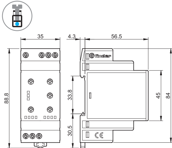
70.41 Bornes à cage
