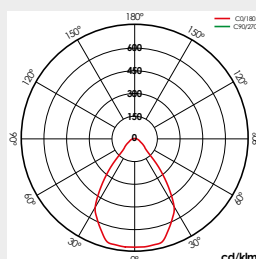
Superficie S069L0P Surface S069L0P Superficie S069L0P Superficie S069L0P
