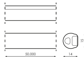
ESQUEMA DE DOBLADO
