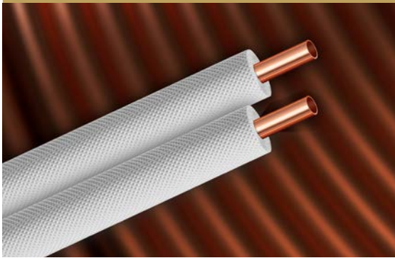
Isolant en polyéthylène réticulé, ignifugé de 10 mm, revêtu d'un film protecteur (épaisseur 50 µm).
